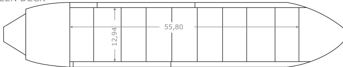
TWEEN DECK
