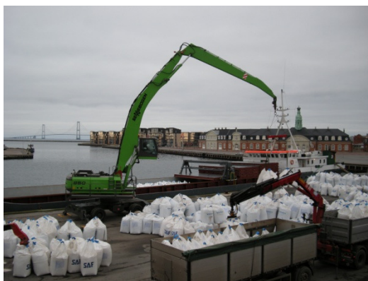
Sennebogen 850
